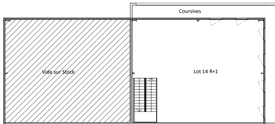
Premier étage
