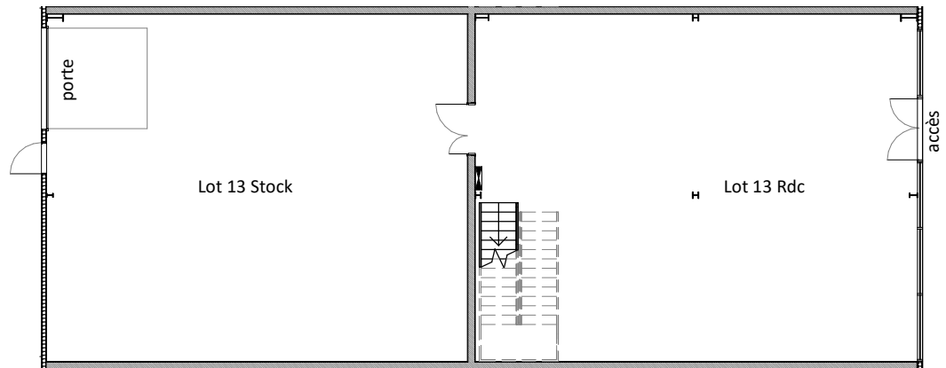
Rez-de-chaussée
